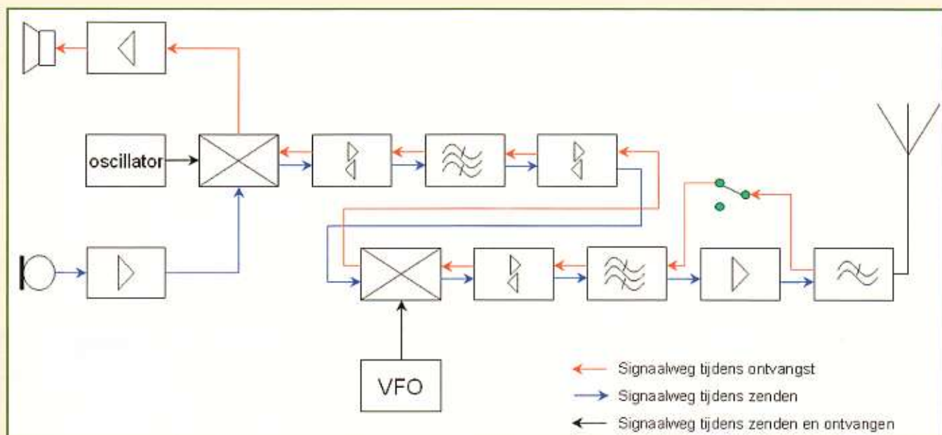
Blok-schema BITX20 compact kleur
